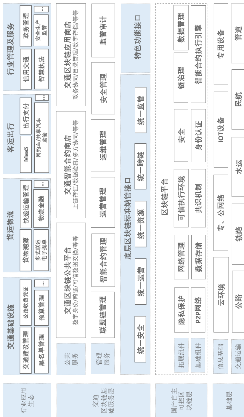
图1 交通运输区块链应用整体架构图
